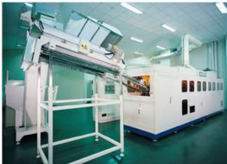
PET耐熱結晶瓶－結晶線 High-Speed Preform Crystallizing Machine
